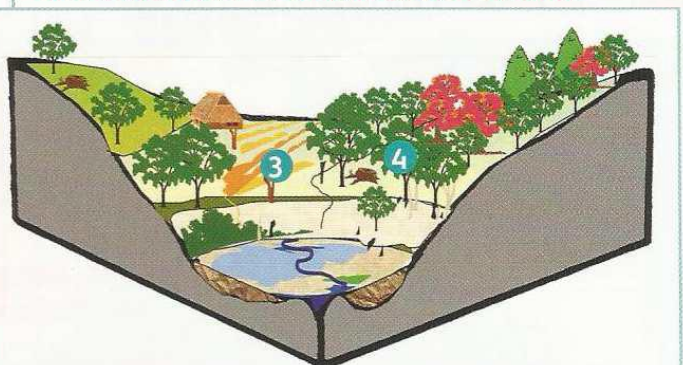
b. Premiers défrichements, disparition de la zone humide et transformation de la forêt
